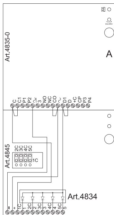
Example of connection with speakerunit Art.4835 Esempio di collegamento con portiere elettrico Art.4835
