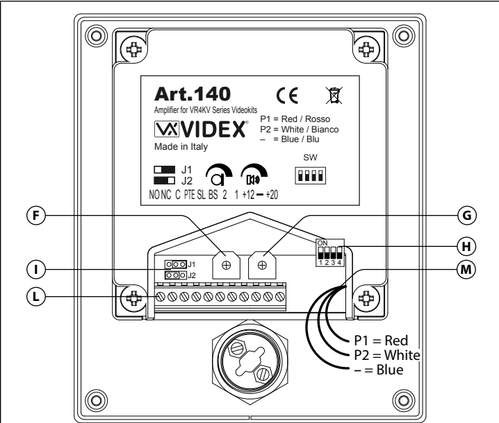
Fig. 2 Back
