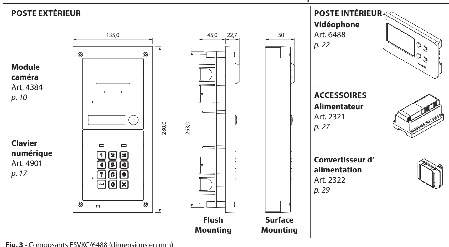
Fig. 3 - Composants ESKV/6488 (dimensions en mm)
